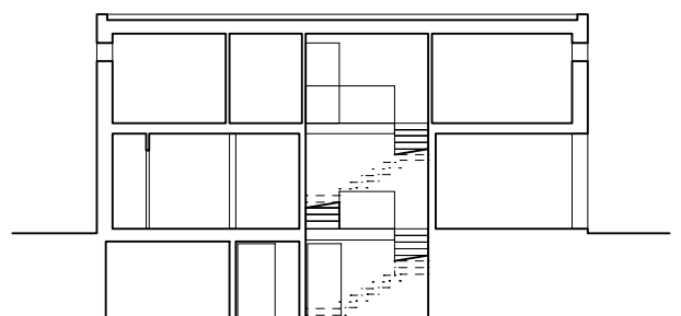
coupe
