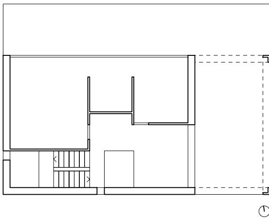
étage 1
