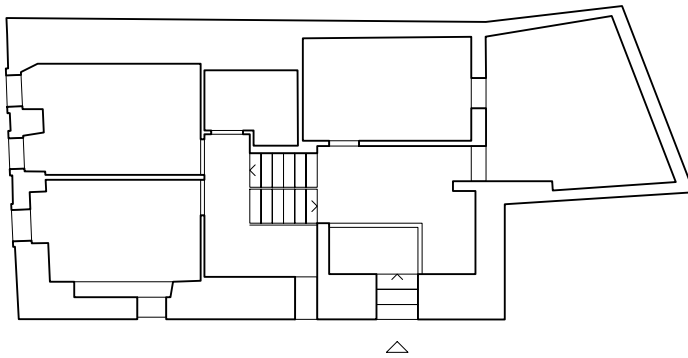
rez inférieur
