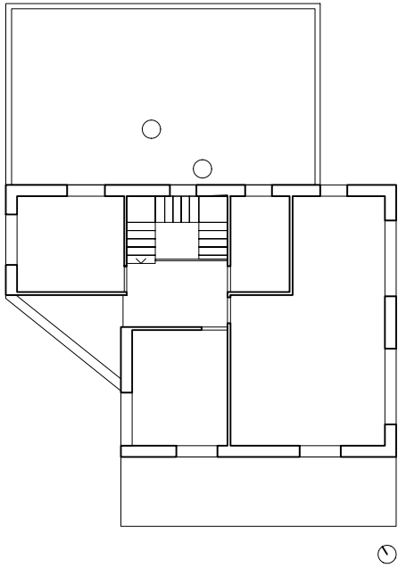
étage
